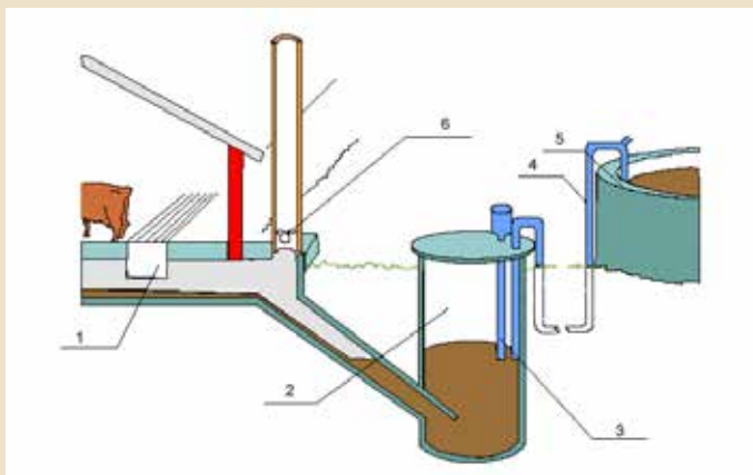
Figura 6.1 - Exemplu de sistem pentru eliminarea deșeurilor lichide 1: canal pentru scurgerea deșeurilor lichide, 2: fosă pentru stocarea intermediară a deșeurilor lichide, 3: pompă, 4: tuburi, 5: rezervor pentru stocarea deșeurilor lichide, 6: ventilație (preluată după Codul de bune practici agricole elaborat de Lituania)
