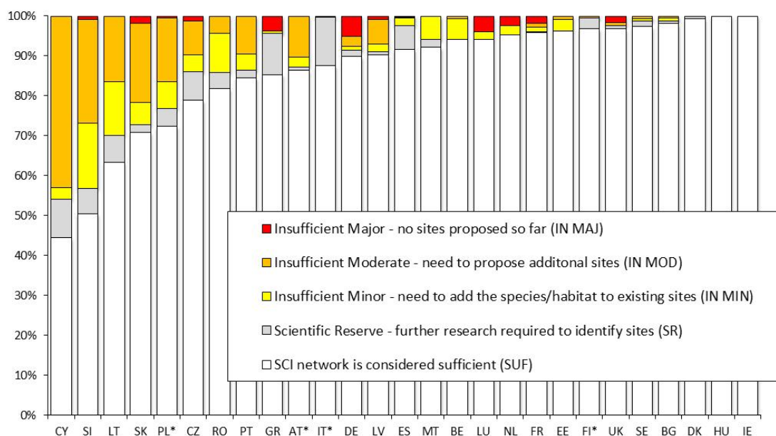
Siturile de importanță comunitară din zona terestră la nivelul UE (sursa: CE - DG Environment)
