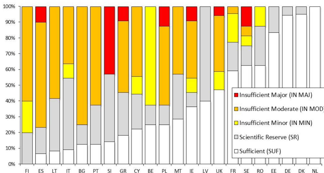
Siturile de importanță comunitară din zona marină la nivelul UE (sursa: CE - DG Environment)
