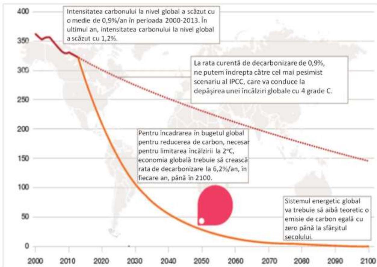
Figura 17: Calea către o stabilizare la 2°C
