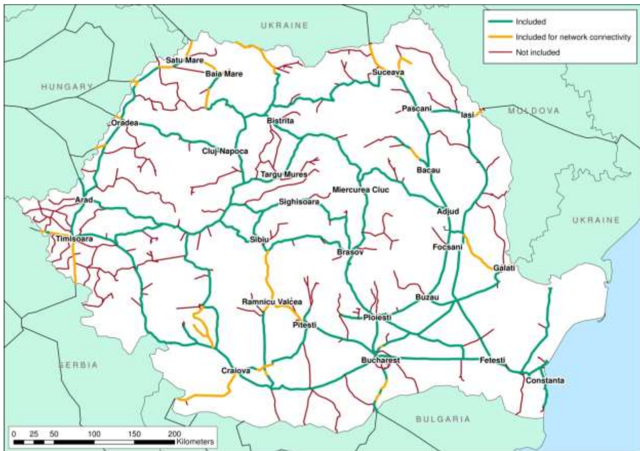
Figura 4. Rețeaua feroviară redusă – propunere MPGT
