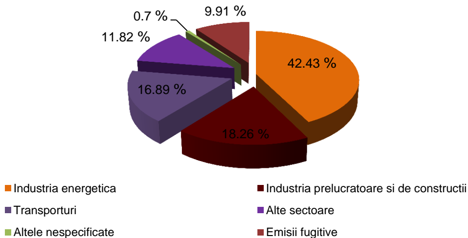
Figura nr. 2-8 Contribuția subsectoarelor de activitate, din cadrul sectorului Energie, la nivelul total al emisiilor de gaze cu efect de seră, la nivelul anului 2011 (sursa: Raportul Inventarului Național al Gazelor cu Efect de Sera, transmis în anul 2013)
