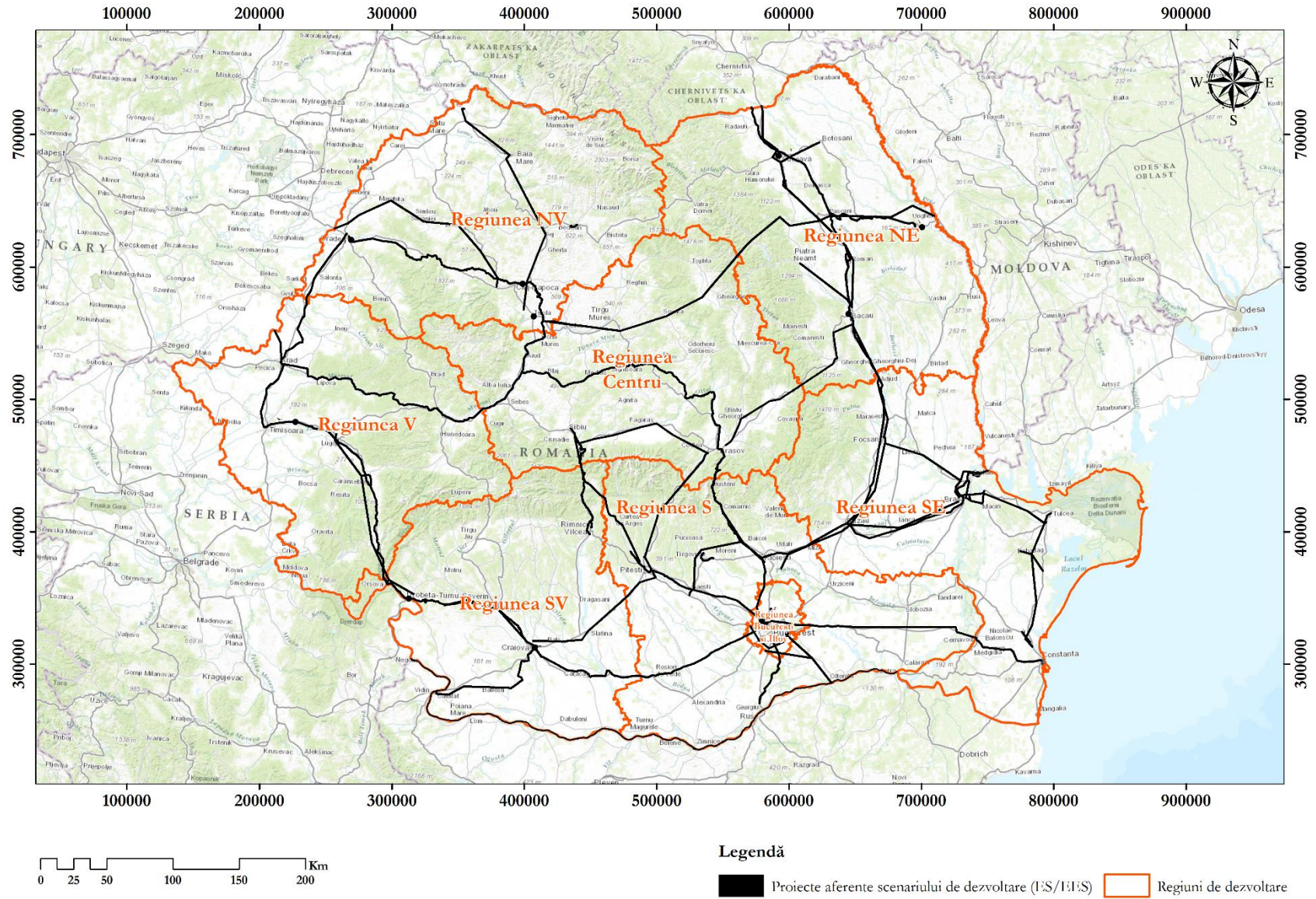
Figura nr. 2-5 Amplasarea proiectelor ce includ lucrări de construcții, cu evidențierea regiunilor de dezvoltare. Conform ultimei versiuni a MPGT (31.08.2014) – scenariul de dezvoltare (ES/EES)
