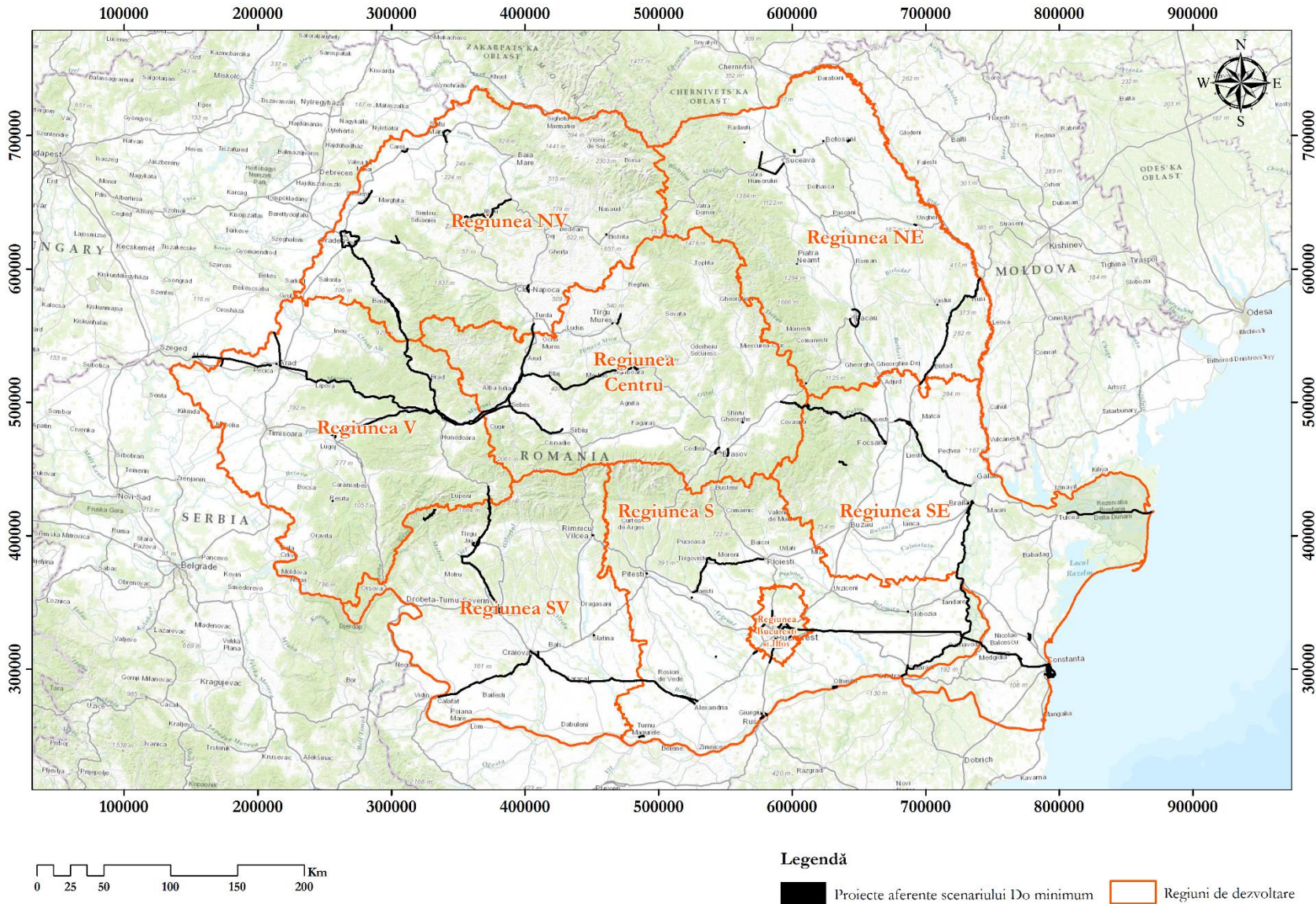
Figura nr. 2-4 Amplasarea proiectelor ce includ lucrări de construcții, cu evidențierea regiunilor de dezvoltare. Conform ultimei versiuni a MPGT (31.08.2014) – scenariul Do minimum
